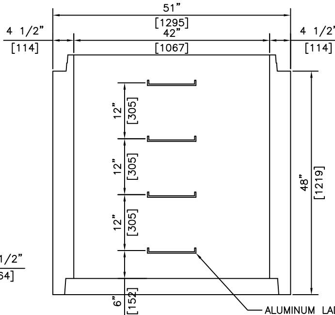
ELEVATION
